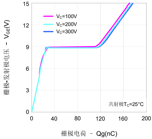
图8. 栅极电荷
