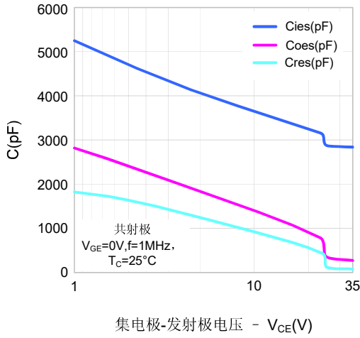
图7. 电容特性
